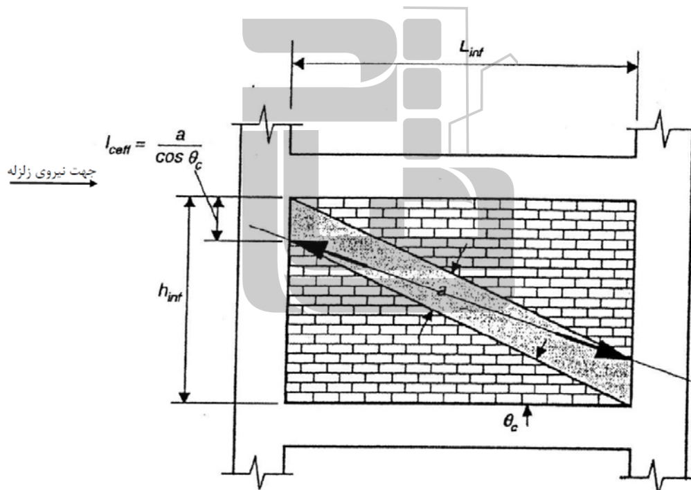
شکل پ ۴۲-۶ - نیروی وارد به ستون از طرف میانقاب
