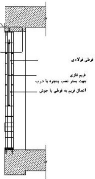
برش A-A
