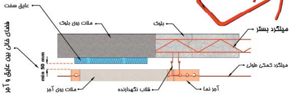
شکل پ-۲۸-۶- نحوه مهار نمای آجری به دیوار پشت
