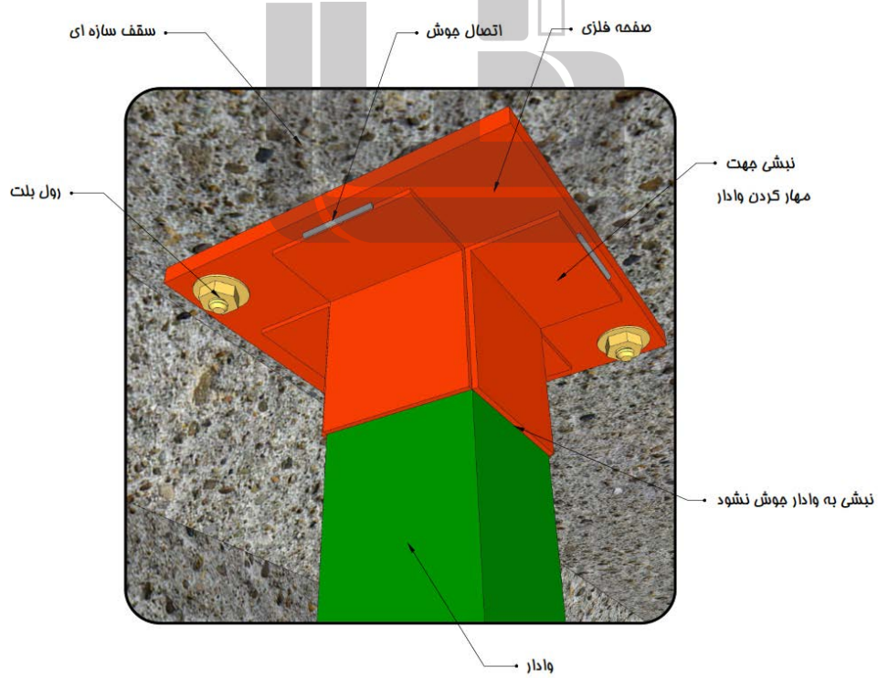
ب- اتصال وادار انتهایی در دیوارهای خارج از قاب به صورت تلسکوپی شکل پ ۶-۶- اتصال وادار به سقف
