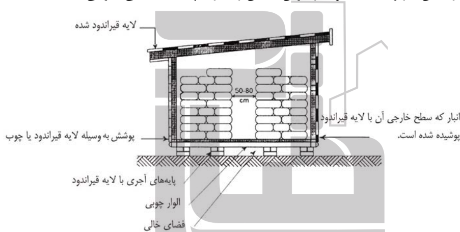
شکل ۲-۷-۲-۸ (ب) انبار کردن سیمان در فضای بسته
