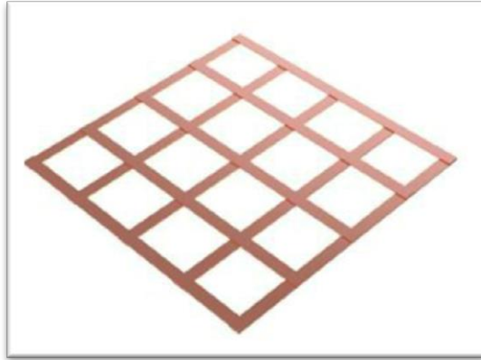
شکل (۲-۱۰): الکتروود تسمه‌ای شبکه‌ای (Lattice) نوعی از صفحه که دارای وزن کمتر و اثری مشابه است.
