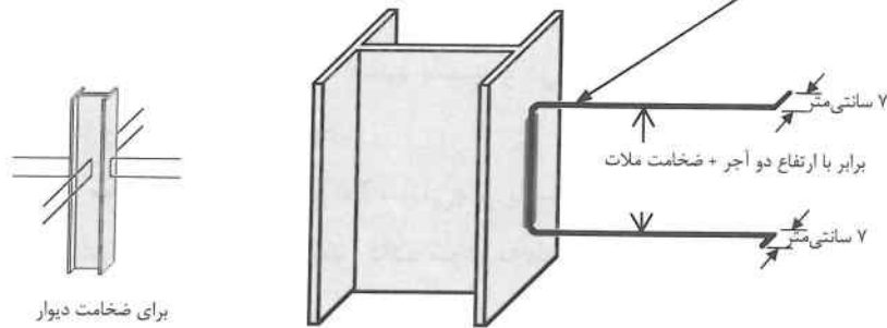
ب- نحوه اتصال ستون فولادی (یا کلاف فولادی) به دیوار آجری
