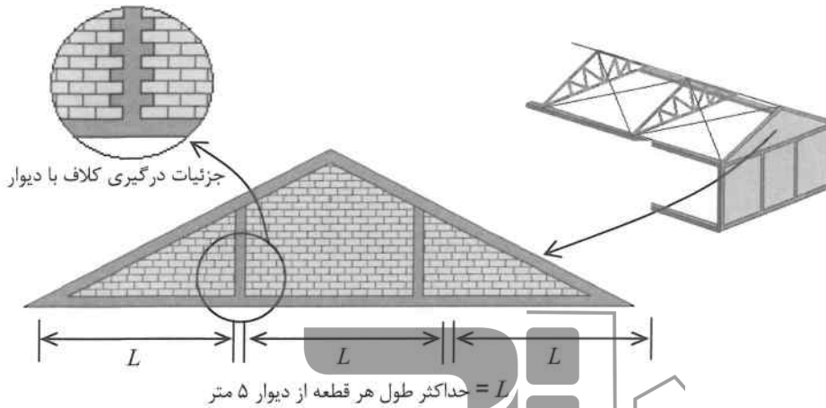
شکل ۲۵-۷ کلاف بندی دیوار انتهایی زیر سقف های شیب دار
