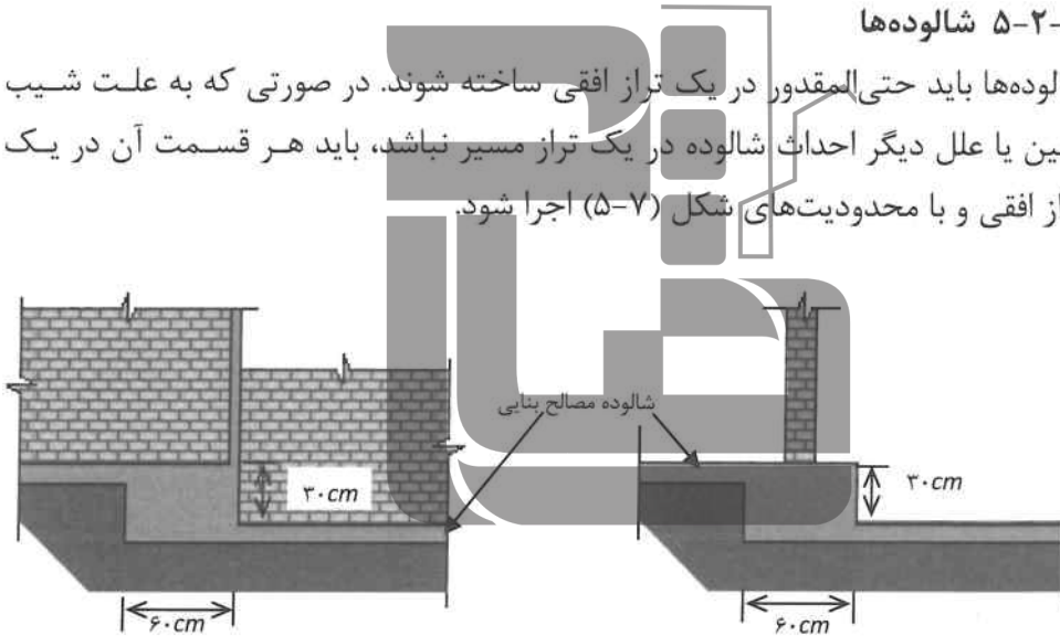
شکل ۵-۷ رعایت ضوابط مربوط به زمین دارای شیب طبیعی
